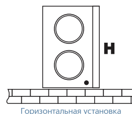
Горизонтальная установка
